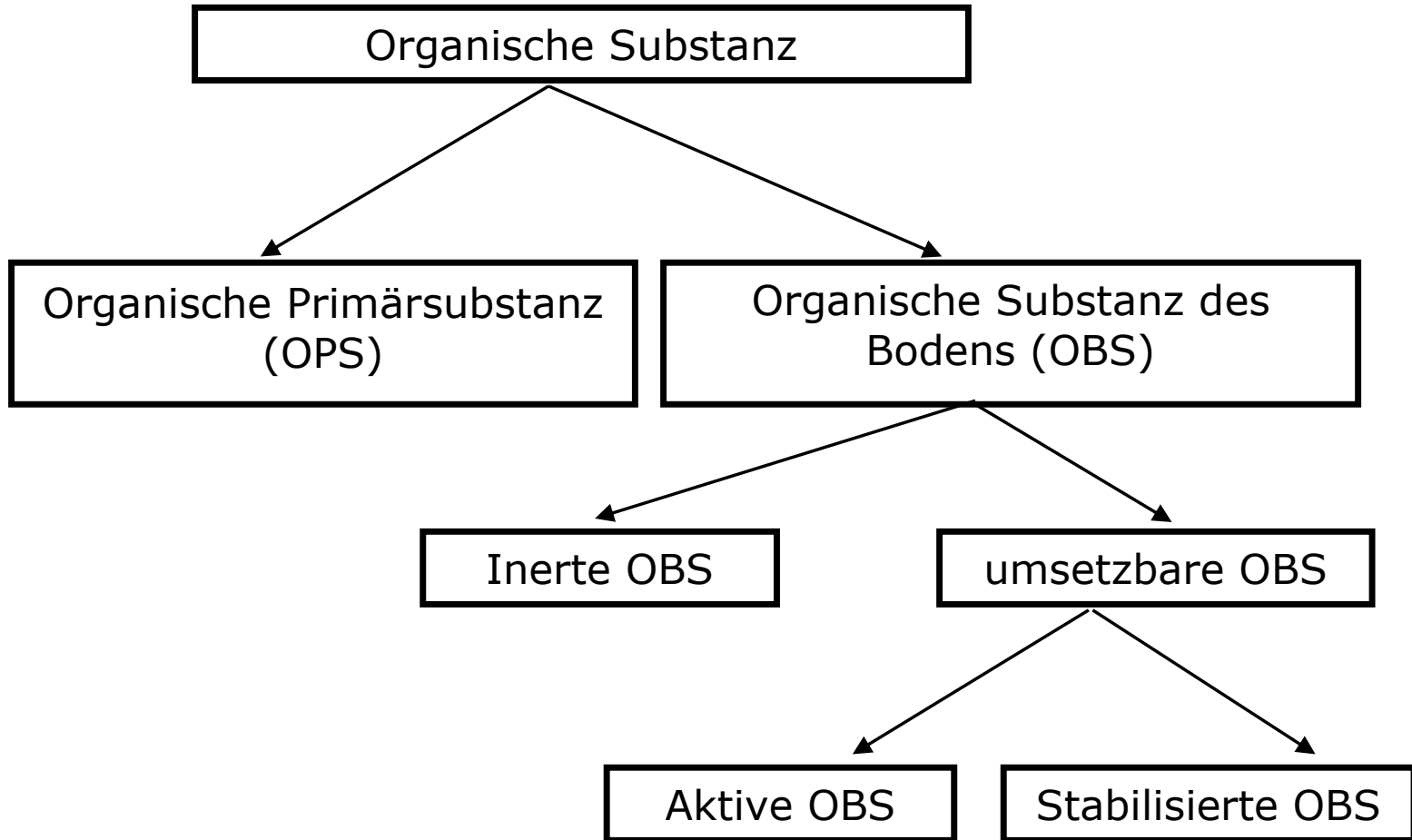
Fractionen der organischen Bodensubstanz (Körschens et al. 1997)
