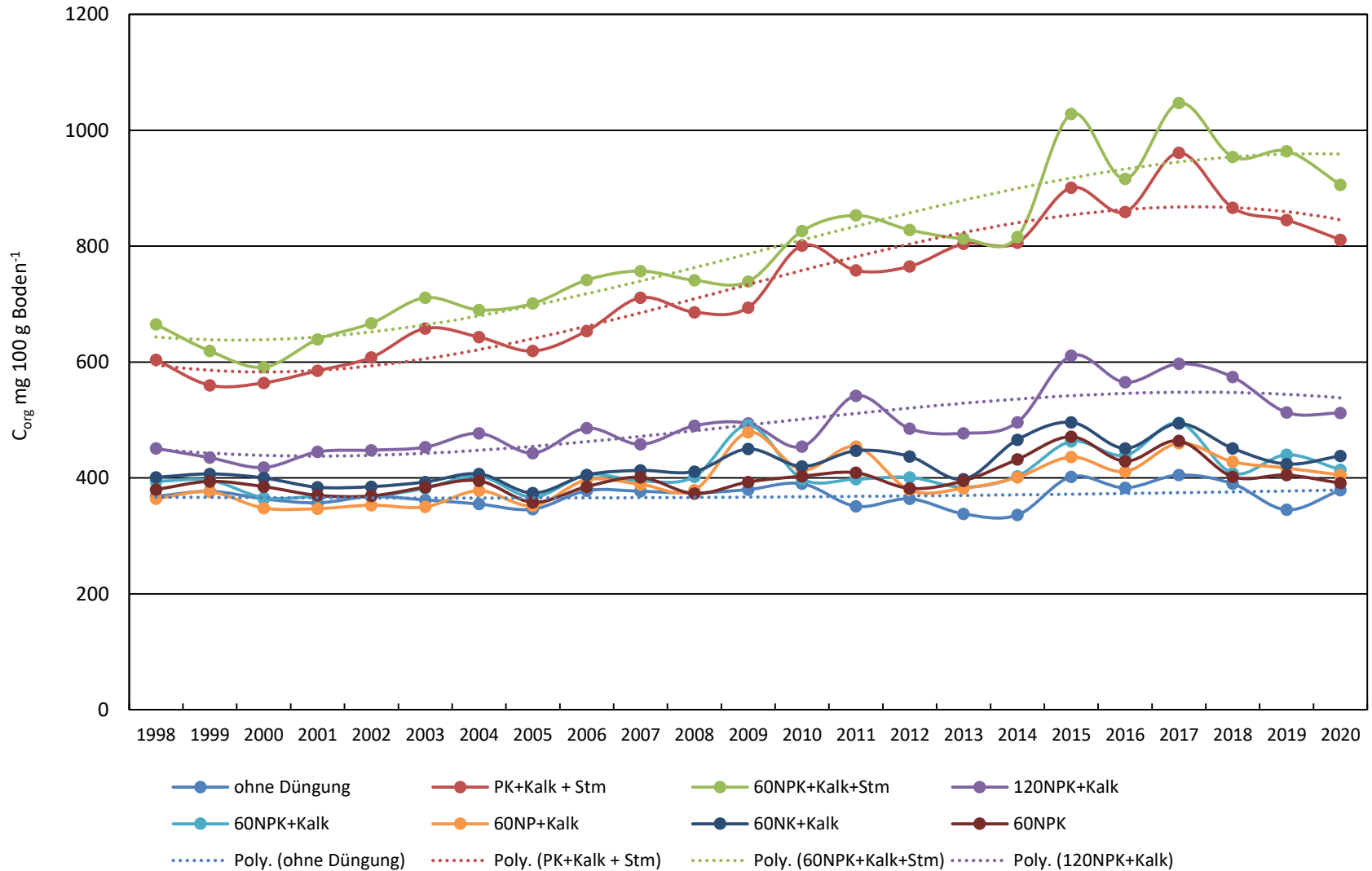
C_{org} -Gehalte Nährstoffmangelversuch Winterroggen Thyrow seit Versuchsbeginn 1998
